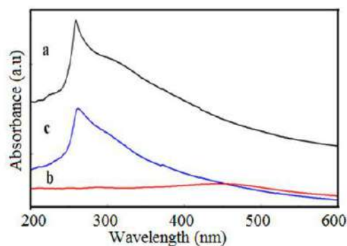
Figure.2: UV spectrum of a) GO b) P-NMPy and c) GO/P-NMPy polymer composite.
