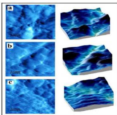
Figure.7:AFM images of a) GO b) P-NMPy c) GO/P-NMPy
